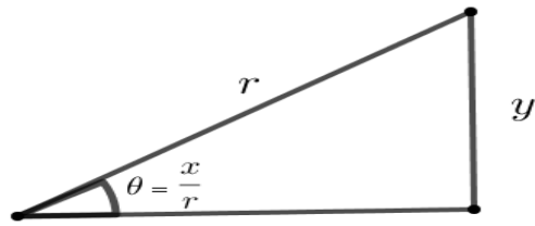
Fig. 4 - Triângulo inscrito no sector circular.
