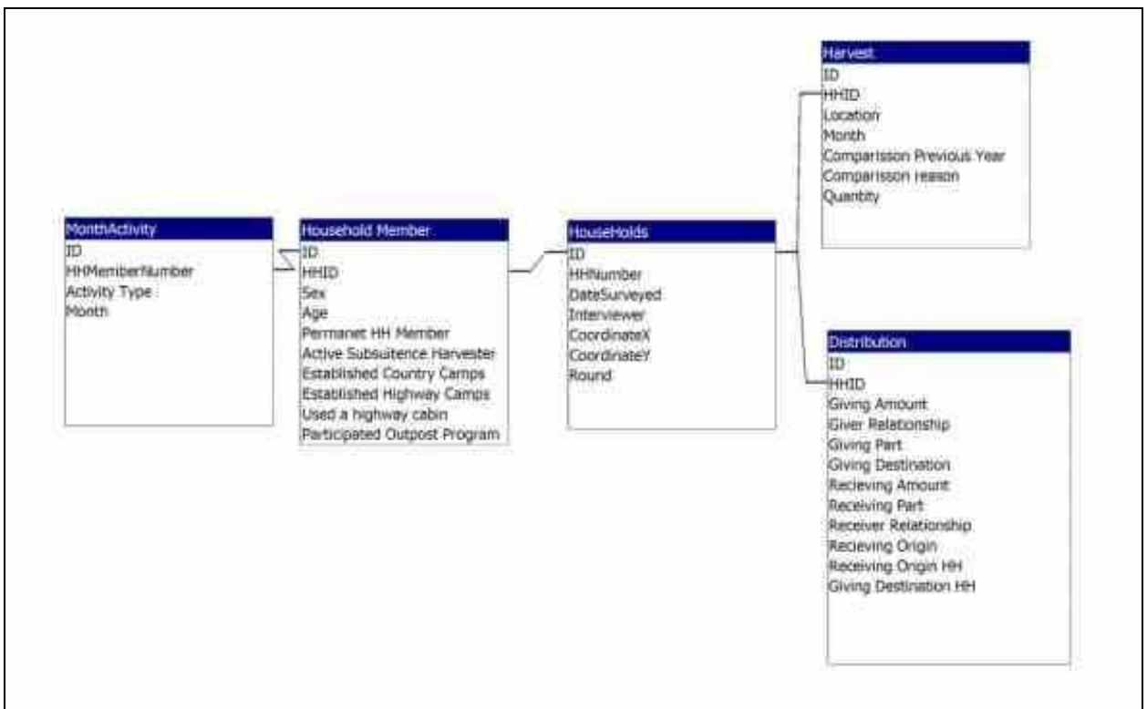
Fig.: Diagrama de la base de datos
