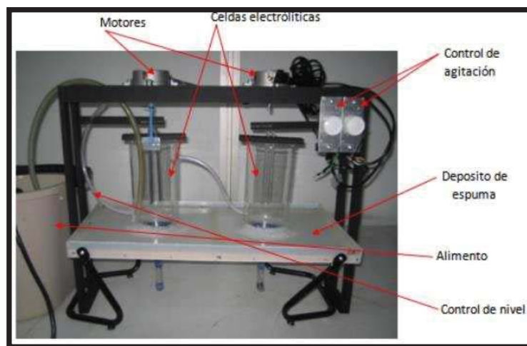
Figura 31: Dispositivo de electro-coagulación flotación. Fte.: Agencia AUPEC (2009).
