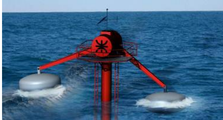
Imagen renderizada del equipo a escala real (Figura 13)
