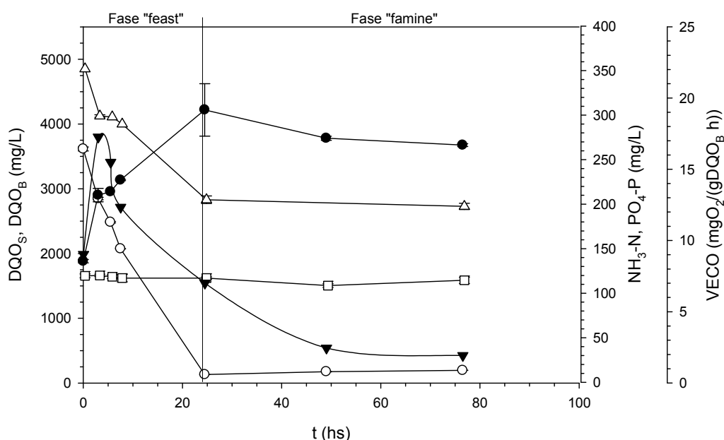
Figura 1. Parámetros químicos de un ciclo de operación del SBR alimentado con medio de cultivo basado en suero de queso. (○) DQO soluble (DQO S , mg/L); (●) DQO de biomasa (DQO B , mg/L); (Δ) Nitrógeno amoniacal (N-NH 3 , mg/L); (□) Ortofosfato (P-PO 4 3- , mg/L); (▼) Velocidad específica de consumo de oxígeno (VECO, mgO 2 /(gDQO B h))
