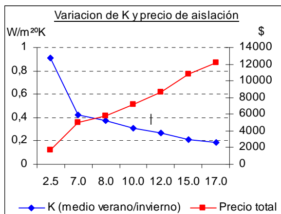
Figura 7: Variación de K y costos para aislación de cubierta
