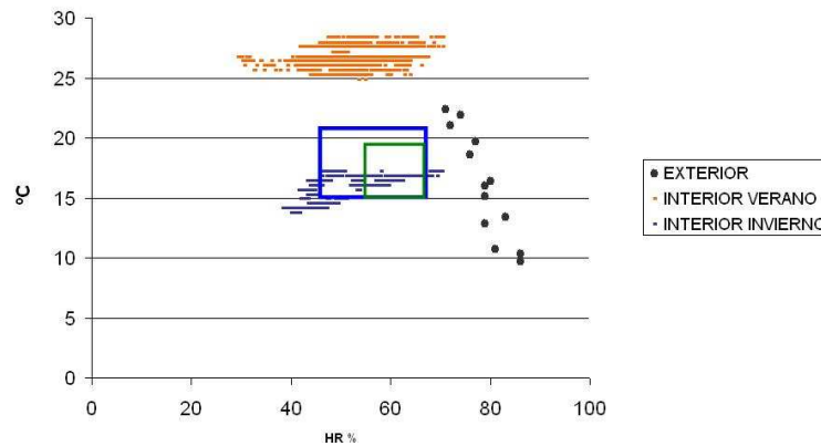
Figura 2 – Datos climáticos relevados en el sitio. Temperatura y HR exterior mensual; temperatura y HR interior de verano; temperatura y HR interior de invierno.
