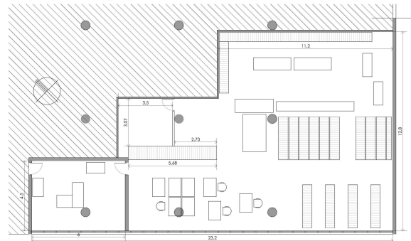
Figura 4: AG - Planta del edificio
