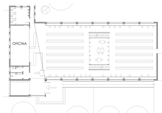
Figura 1: BCI - Planta del edificio
