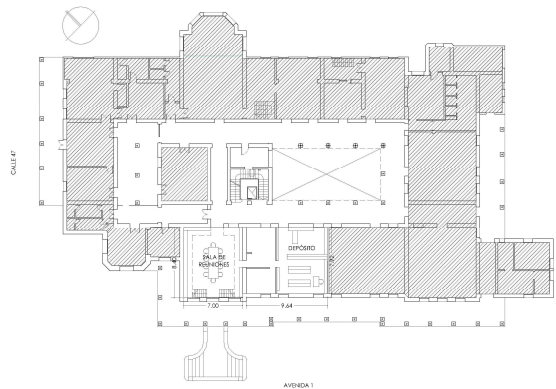
Figura 2: BHDC - Planta del edificio
