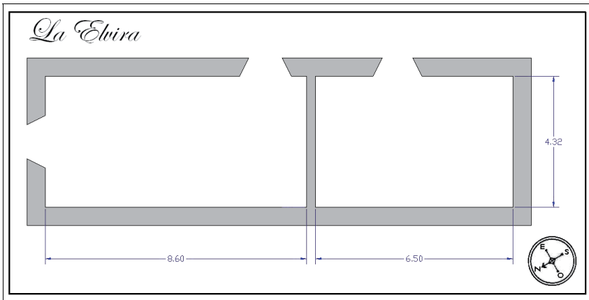
Figura 9. Plano de la estructura original de la casa, de acuerdo a los datos recopilados. Medidas en metros
