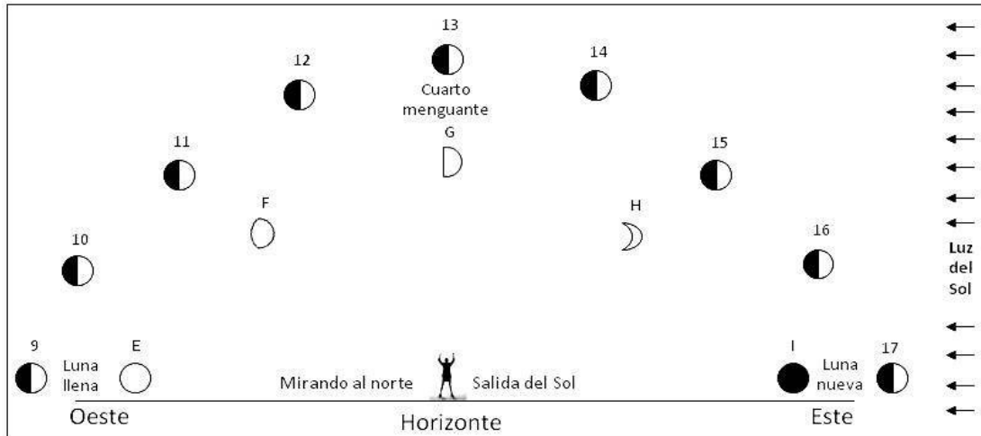
6 Figura 3. Esquema topocéntrico explicativo de la fase menguante de la Luna para un observador ubicado en 7 latitudes medias del hemisferio sur (Galperin, 2016).
