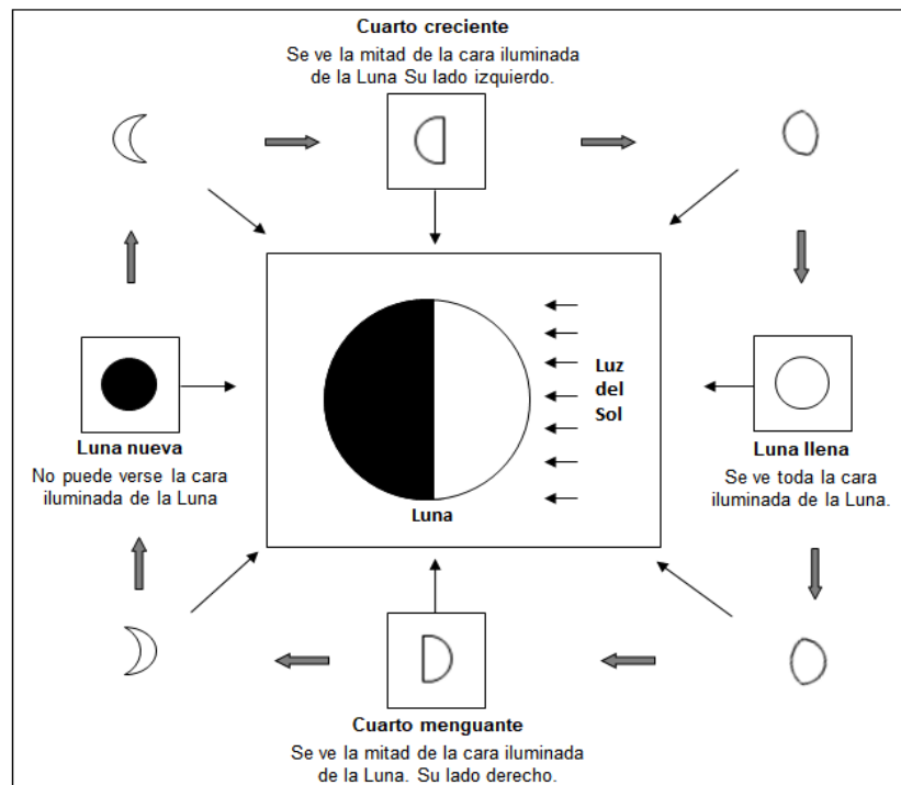
22 Figura 1. Esquema explicativo de las fases lunares para el hemisferio sur: cómo se observa una esfera iluminada 23 por la mitad (que representa la Luna) desde distintos puntos de vista (Galperin, 2016).
