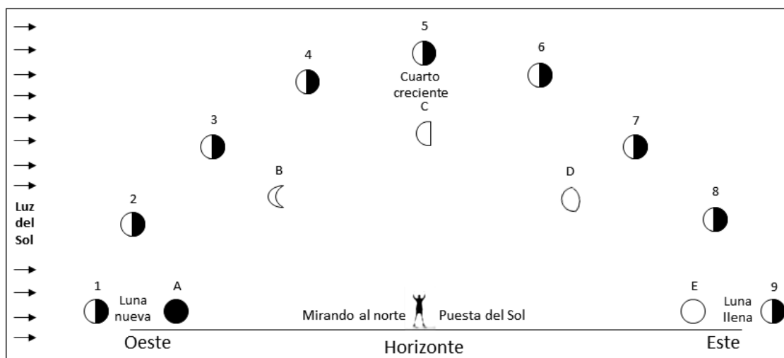
13 Figura 2. Esquema topocéntrico explicativo de la fase creciente de la Luna para un observador ubicado en 14 latitudes medias del hemisferio sur (Galperin, 2016).
