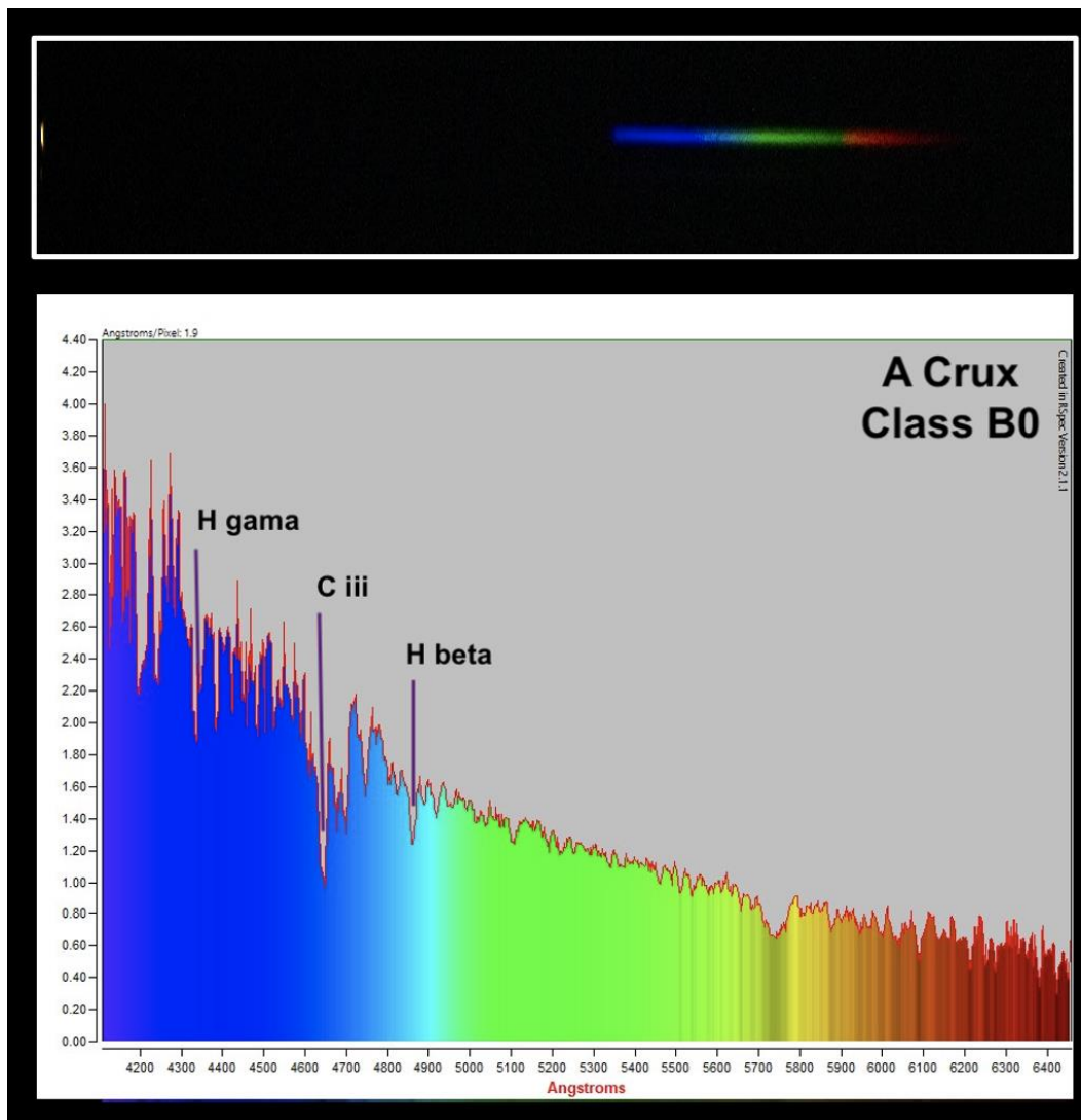
Figura 4. Espectro obtenido de Alfa Cruz.
