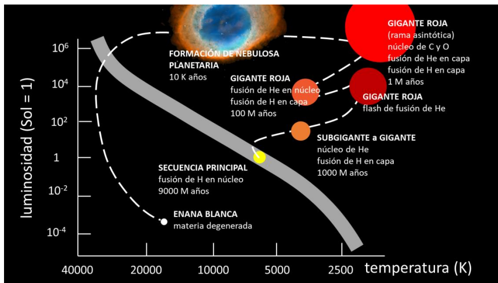
Figura 4. La evolución del Sol en el diagrama H-R.
