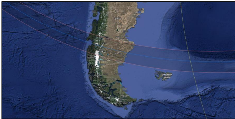
Figura 11. Trayectoria del próximo eclipse anular de Sol visible en la Patagonia argentina el 2 de octubre de 2024.
