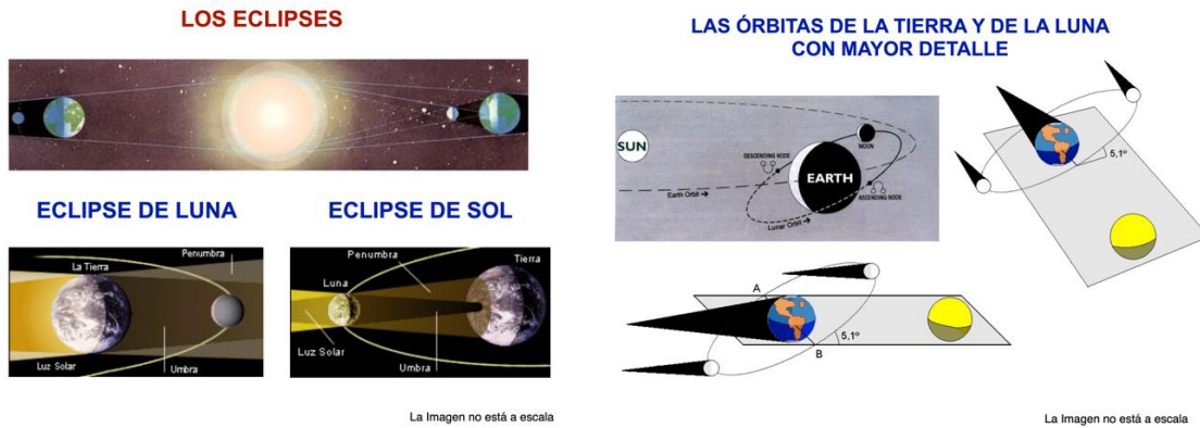
Figura 1. Izquierda: esquema de las posiciones del Sistema Sol-Tierra-Luna en los eclipses. Derecha: detalle de la inclinación de las órbitas del Sistema Sol-Tierra-Luna
