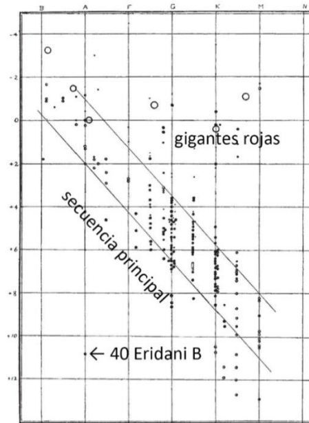
Figura 3. Diagrama original de magnitud absoluta vs clase espectral, adaptado de Russell (1914).
