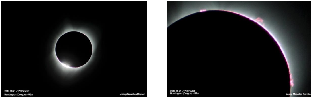
Figura 8. Perlas de Baily y Anillo de diamante (izquierda) y protuberancias visibles (derecha) en el eclipse total de Sol del 21 de agosto de 2017 observado en Huntington (Oregon, USA).
