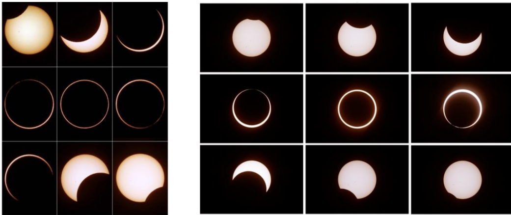
Figura 3. Izquierda: secuencia del eclipse anular del 26 de febrero de 2017 observado en Sarmiento (Chubut, Argentina). Derecha: secuencia del eclipse anular del 14 de octubre de 2023 observado en Albuquerque (New México).
