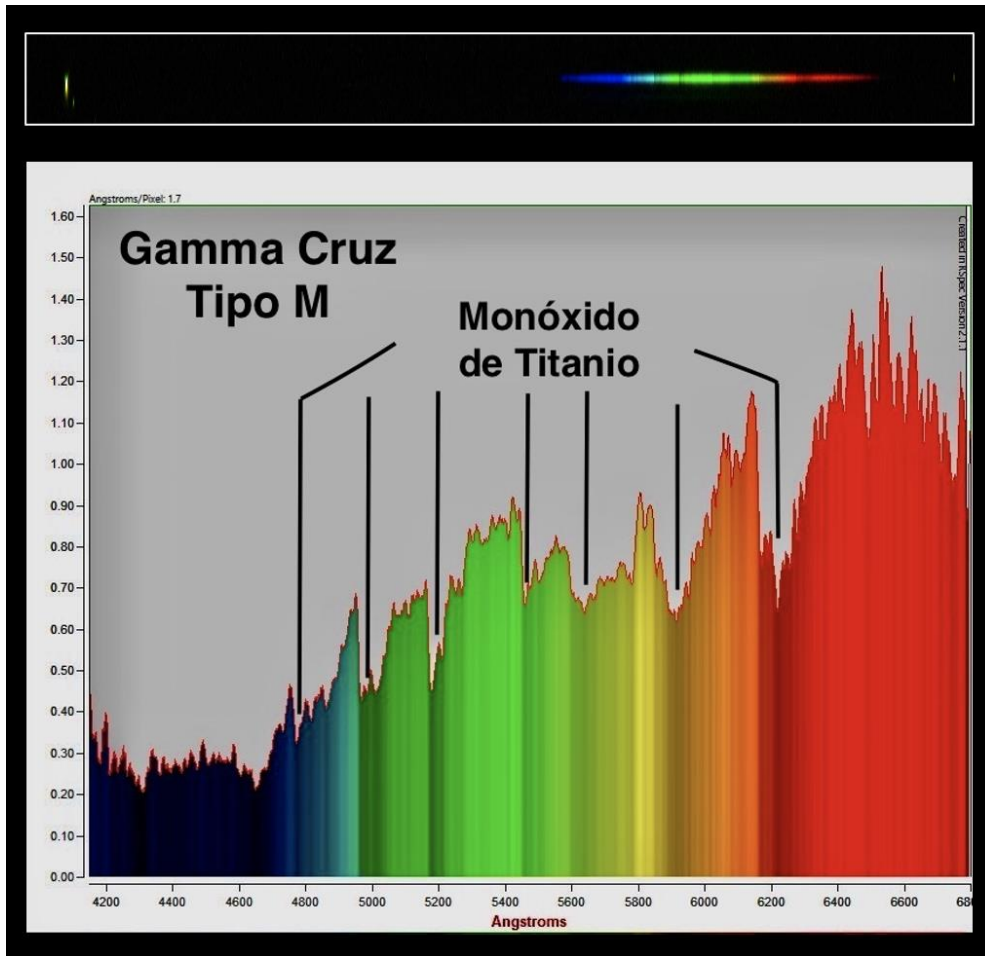
Figura 6. Espectro obtenido de Gama Cruz
