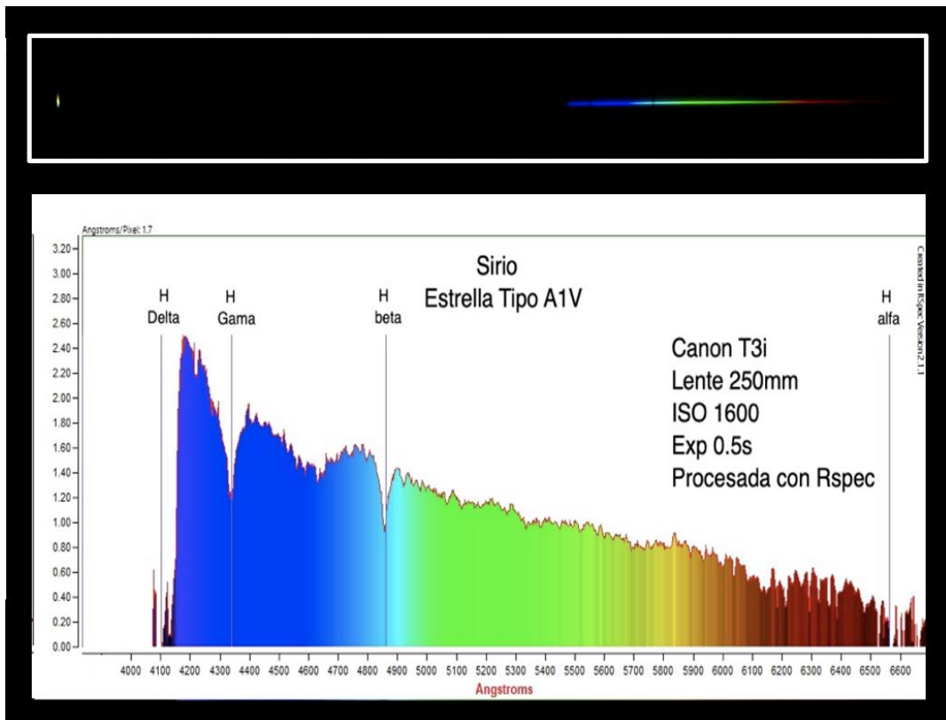
Figura 5. Espectro obtenido de Sirio.
