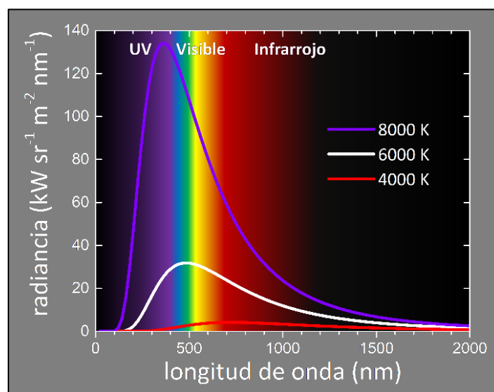
Figura 2. Radiancia espectral de un cuerpo negro, para tres temperaturas (indicadas en kelvins).
