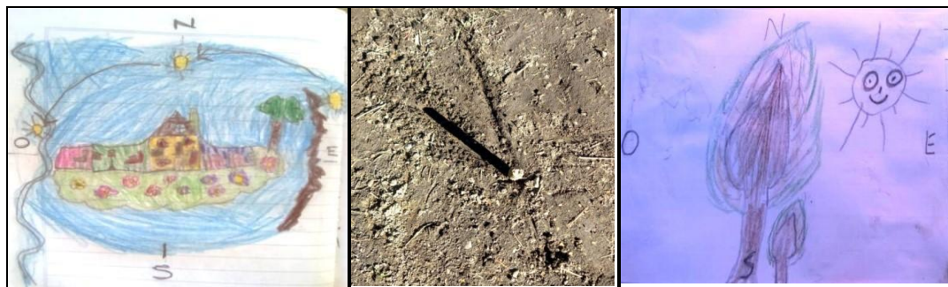
Figura 3. Registros del cambio diario de posición del Sol en el cielo.
