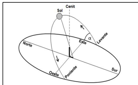
Figura 1. Descripción del movimiento diario del Sol en latitudes medias del hemisferio sur.
