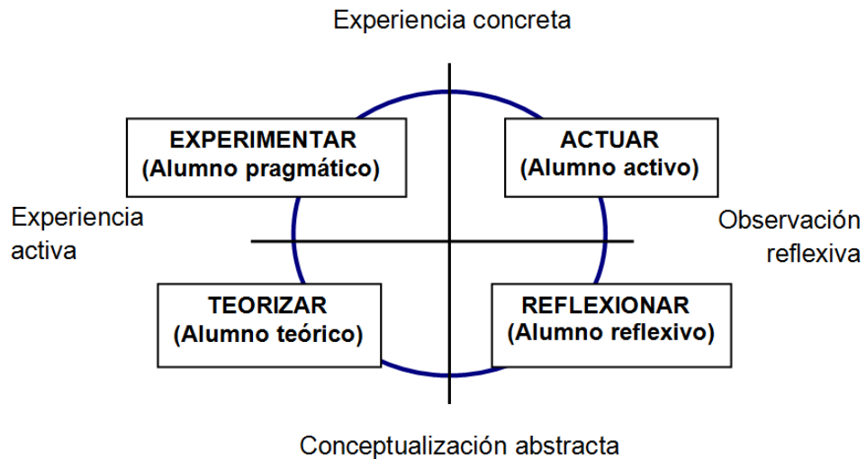
Figura 8: Esquema gráfico del Ciclo de Kolb (1984)
