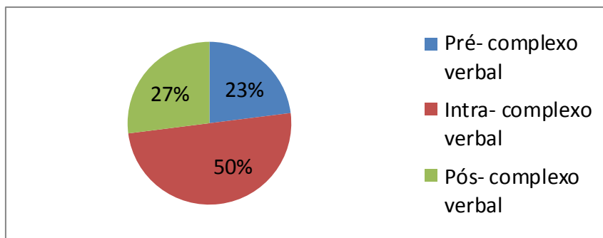
Gráfico 1: Resultados gerais
