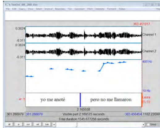
Gráfico 4
