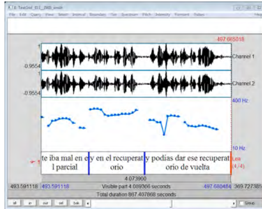
Gráfico 1
