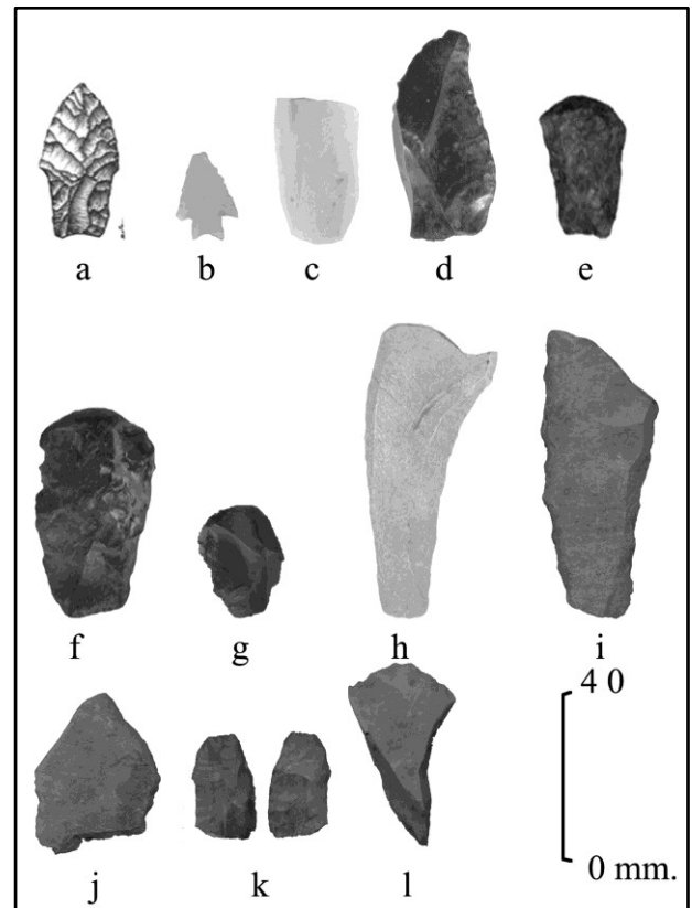
Figura 5. Material lítico de Lago Cástor 1. a) Punta de proyectil Fell IV hallada por F. Bate en 1968, b-l) segunda campaña, b) punta de flecha Fell V, c-d) cuchillos, e-g) raspadores, h-j) raederas, k-l) de función no identificada.
