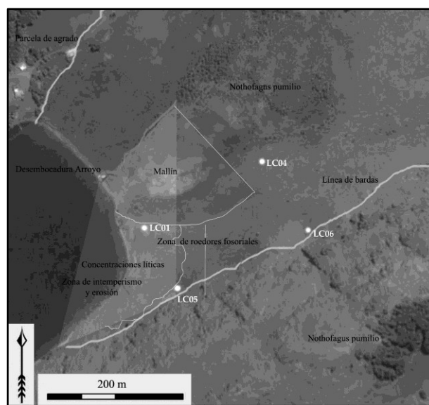
Figura 1. Imagen Landsat indicando localización de concentraciones líticas respecto al área de intemperismo y erosión, relictos de N. Pumilio , línea de bardas, humedal tipo mallín y disturbios por madrigueras de Ctenomys coyhaiquensis (cf. Sade y Pérez 2011: 271).
