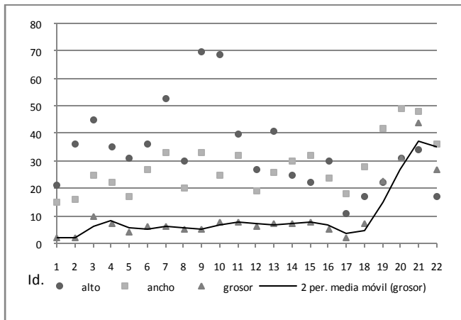
Figura 3. Tendencias métricas (mm.) de los instrumentos de Lago Cástor 1. Campaña del año 2008.
