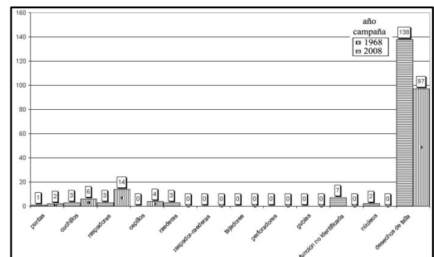
Figura 2. Frecuencia de funcionalidades del instrumental lítico. Campañas de los años 1968 y 2008.
