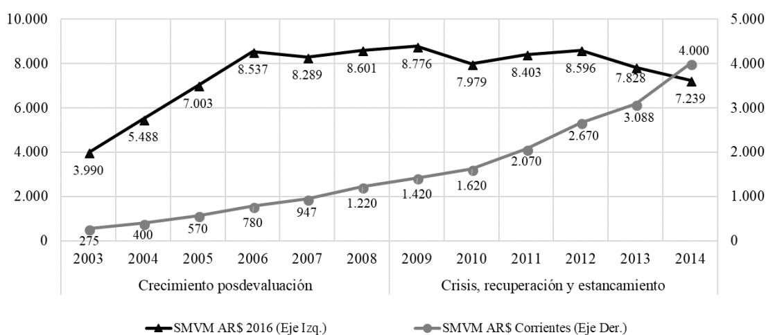
Gráfico 1.6. Evolución del salario mínimo, vital y móvil promedio anual. Argentina, 2003-2014
