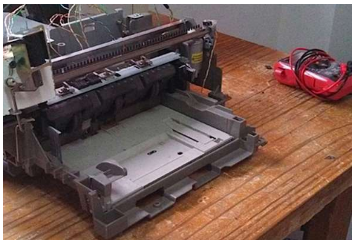
Figura 1. Primer prototipo de impresora braille (Openbraille, 2014)
