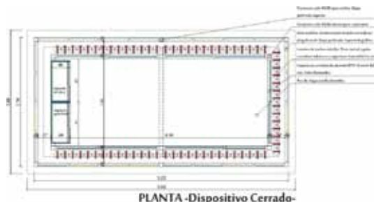
Figura 5. Planta neutra DU
