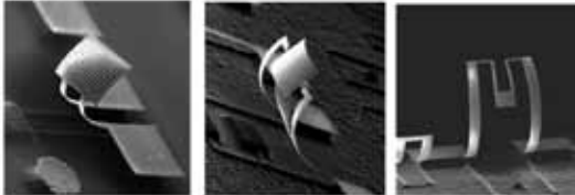
FIGURA 10: Micro-espelhos de TiNi que são comandados através do EMF
